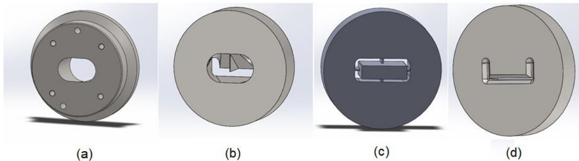
Figure 2.3 (a) Adapter plate; (b) Transition plate; (c) Spider plate; (d) Die plate.
