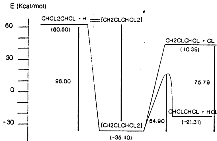
ENERGY DIAGRAM : CHCl 2 CHCl + H (a)
