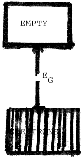
Fig. 1A INSULATOR
