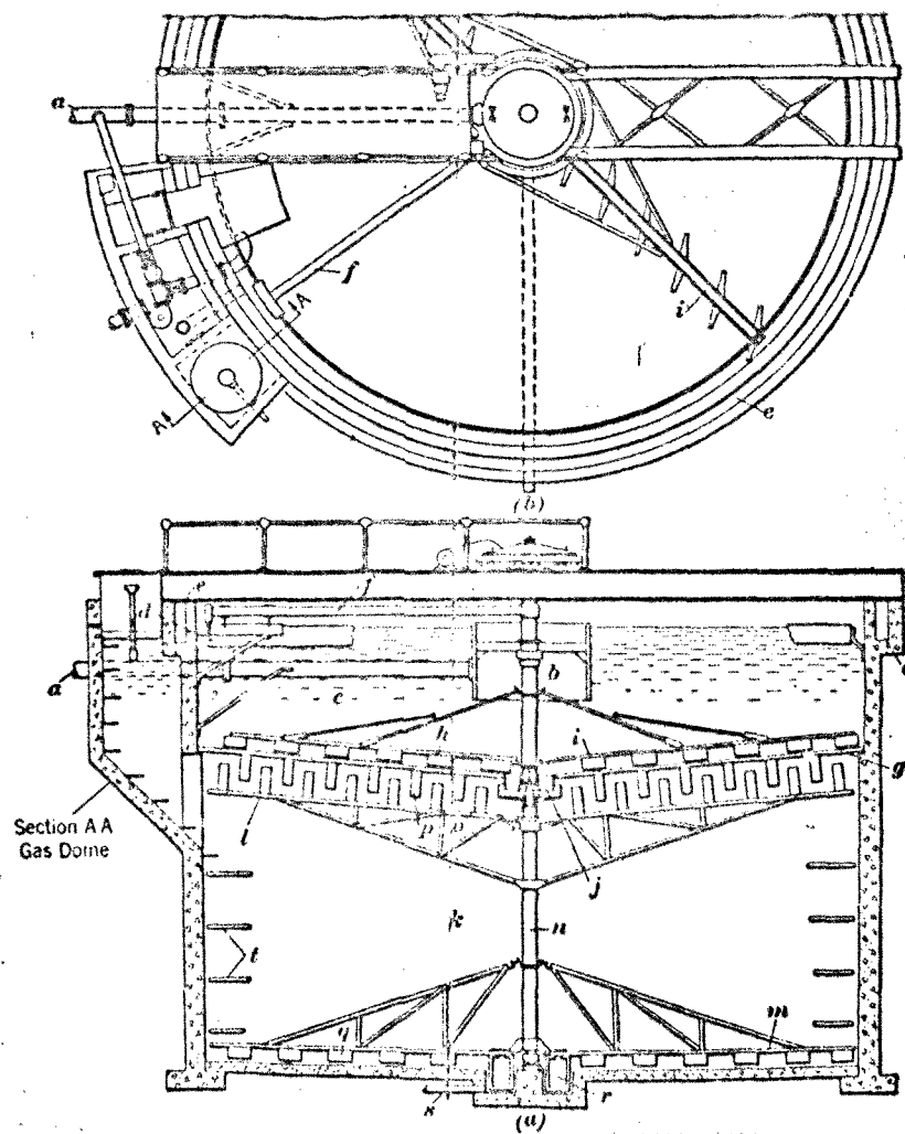
Fig. 5. The Clarigester.
